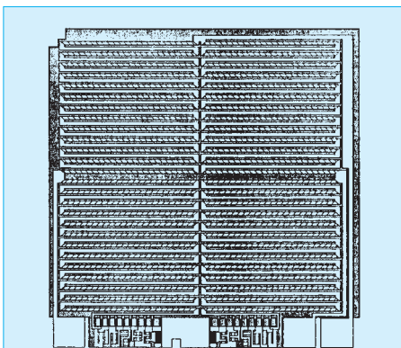
Bild 1: Struktur des KMZ10A1-Chips mit mäanderförmig geführten Leiterbahnen aus Permalloy, goldstreifendurchsetzt, in einer Vollbrücke (Philips, Technische Informationen).
