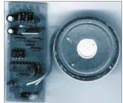
Bild 4: Ansicht des Durchgangsprüfers (hier mit einem Lautsprecher als Signalgeber)
