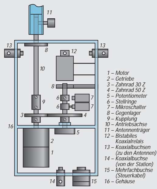
Bild 2: So oder ähnlich sieht der Eigenbau-Rotor aus
