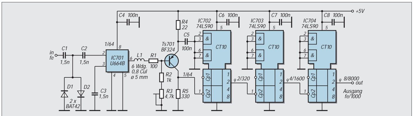
Bild 17: Vorteiler f_e/1000
