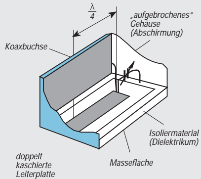
Bild 3: Ansicht eines mit doppelkaschiertem Leiterplattenmaterial aufgebauten Stripline-Leitungskreises. Die Ankopplung kann – wie im Text beschrieben – über eine Koaxialbuchse erfolgen.
