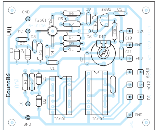
Bild 16: Bestückung der Platine „Eingangsverstärker“
