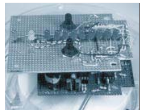
Bild 8: Der Aufbau wurde mittels Lochrasterplatten vorgenommen.
