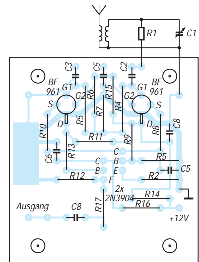
Bild 4: Bestückungsplan
