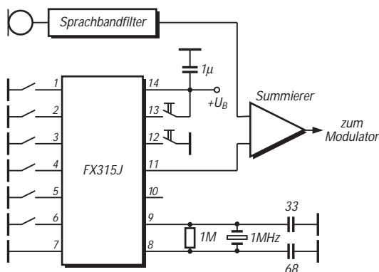
Bild 2: Anwendungsschaltung ohne Besonderheiten
