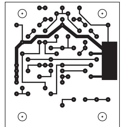
Bild 3: Platinenlayout
