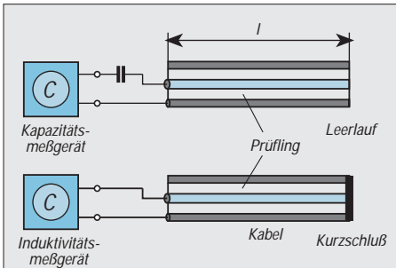
Bild 2: Die Kapazität des Kabels mißt man am leerlaufendem Leitungsstück; die Induktivität am kurzgeschlossenen Leitungsstück.
